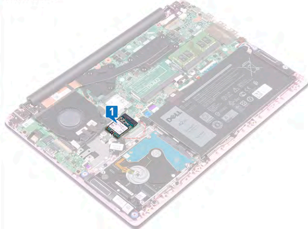
M.2 2230
