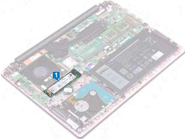
M.2 2280
